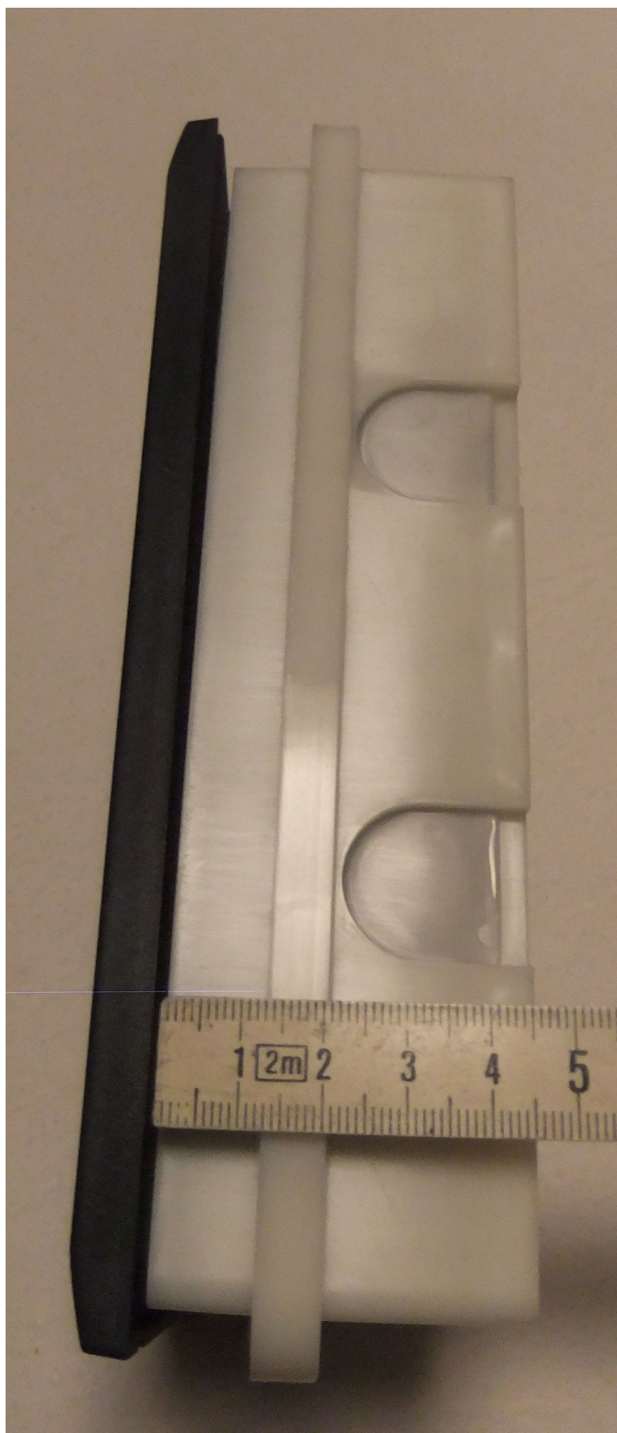
Achterzijde – inbouw - diepte freeswerk – met meegeleverd inbouwbakje
