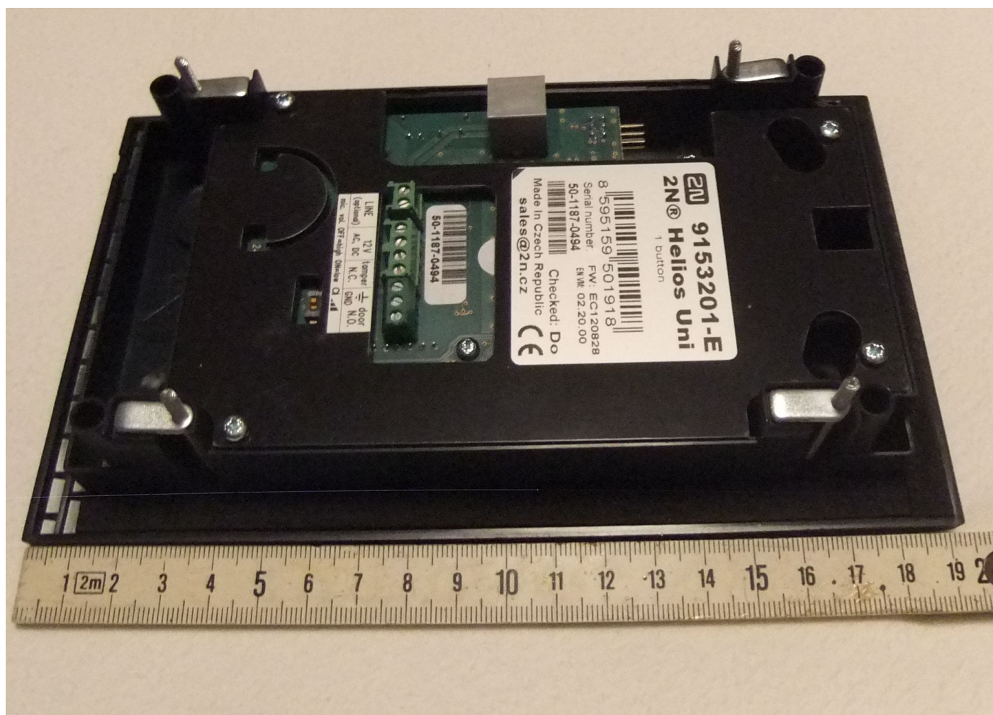
Achterzijde – maximale hoogte buitenwerks
