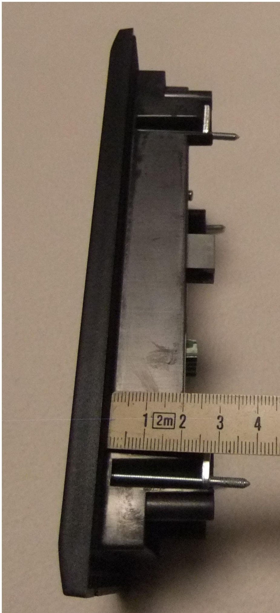
Achterzijde – inbouw - diepte freeswerk – zonder inbouwbakje
