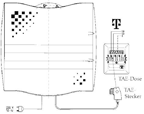
Aufputzinstallation
