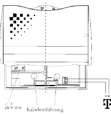
Unterputzinstallation
